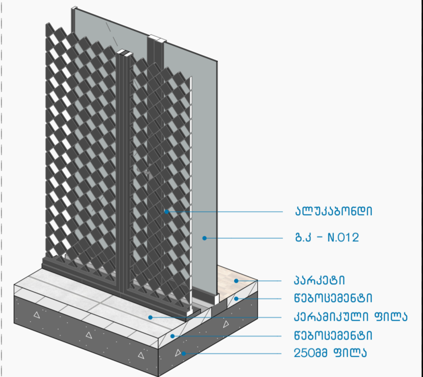
კვანძი N48 1:30
