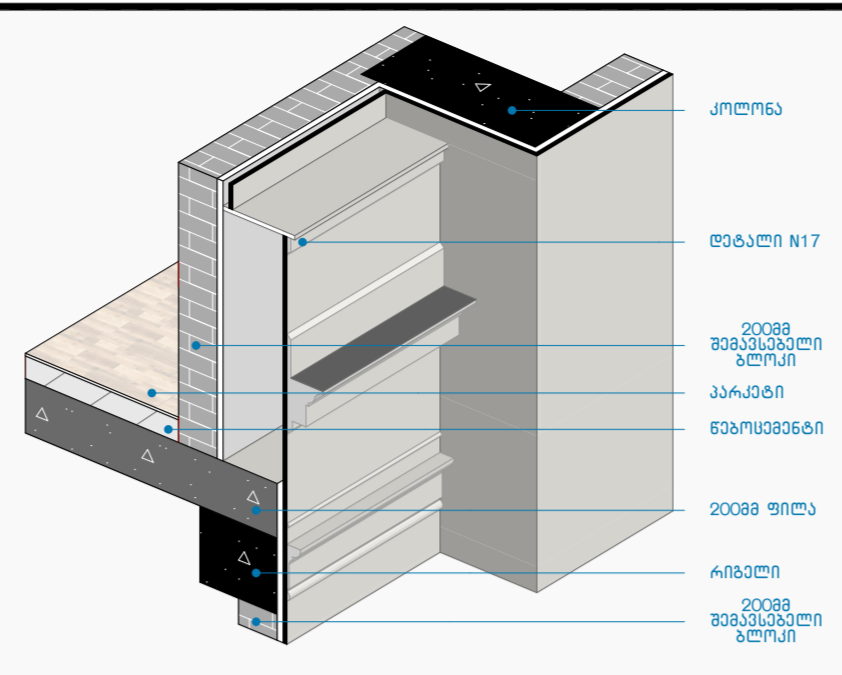
კვანძი N29 1:30
