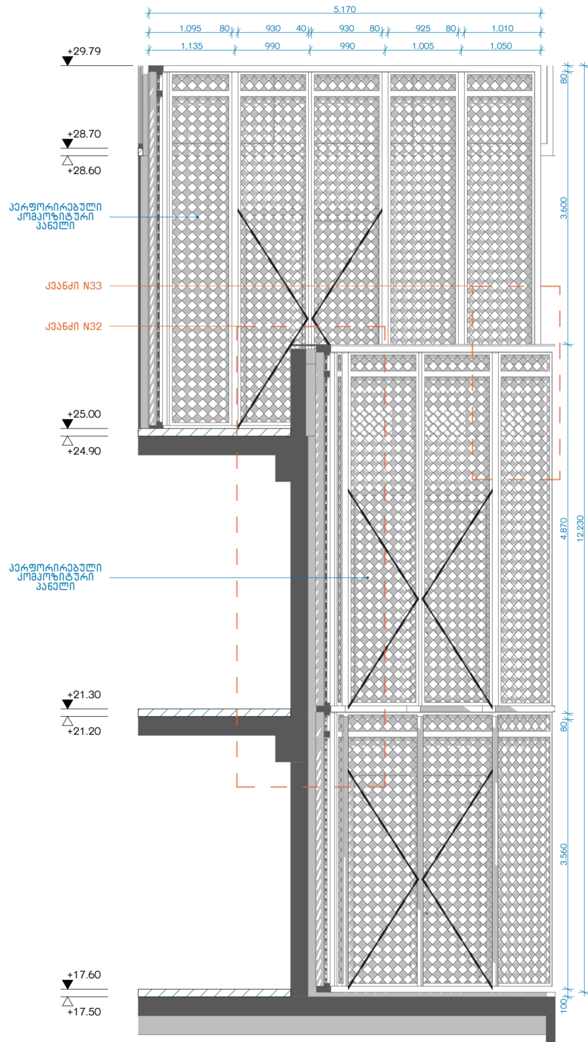
ფასადი 1-8 / ფ-19
