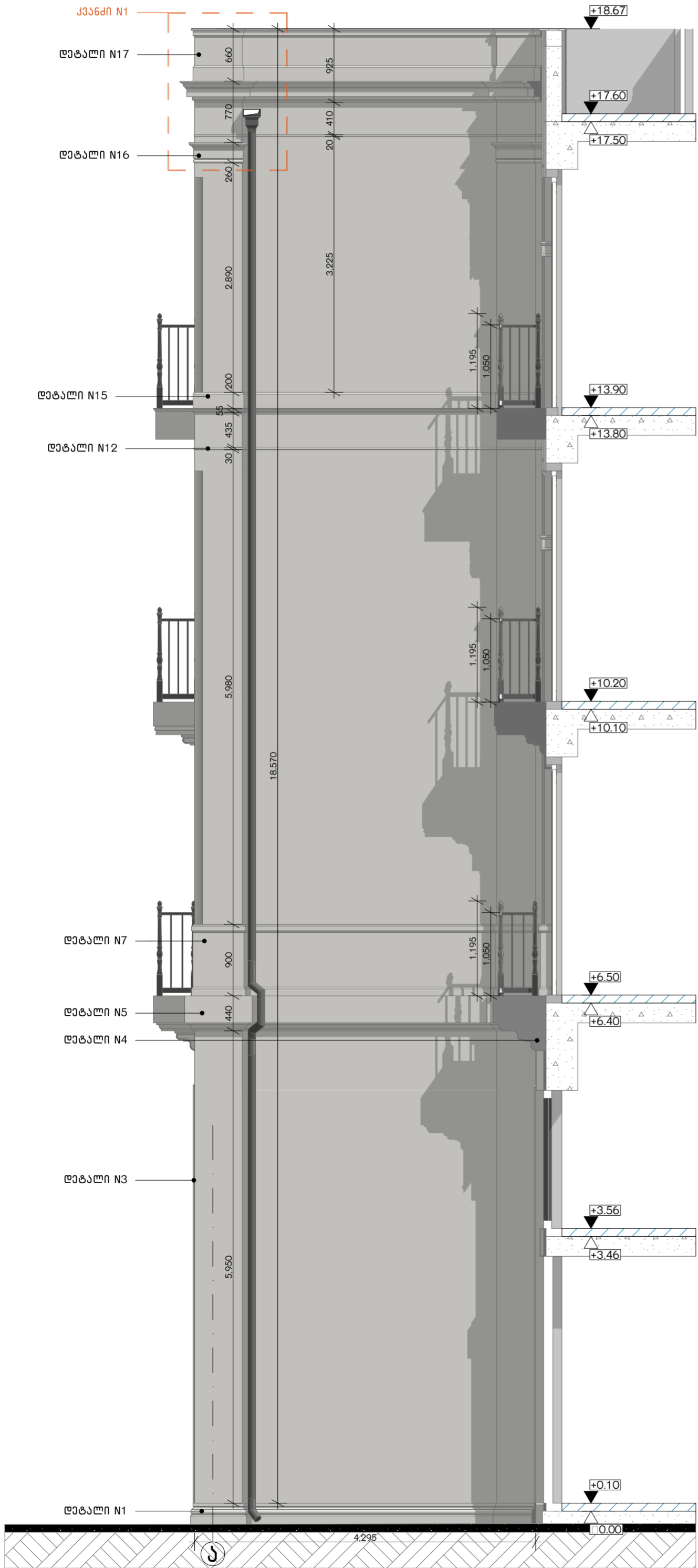
ფასადი 1-8 ლიქებში / ფ-2 1:50
