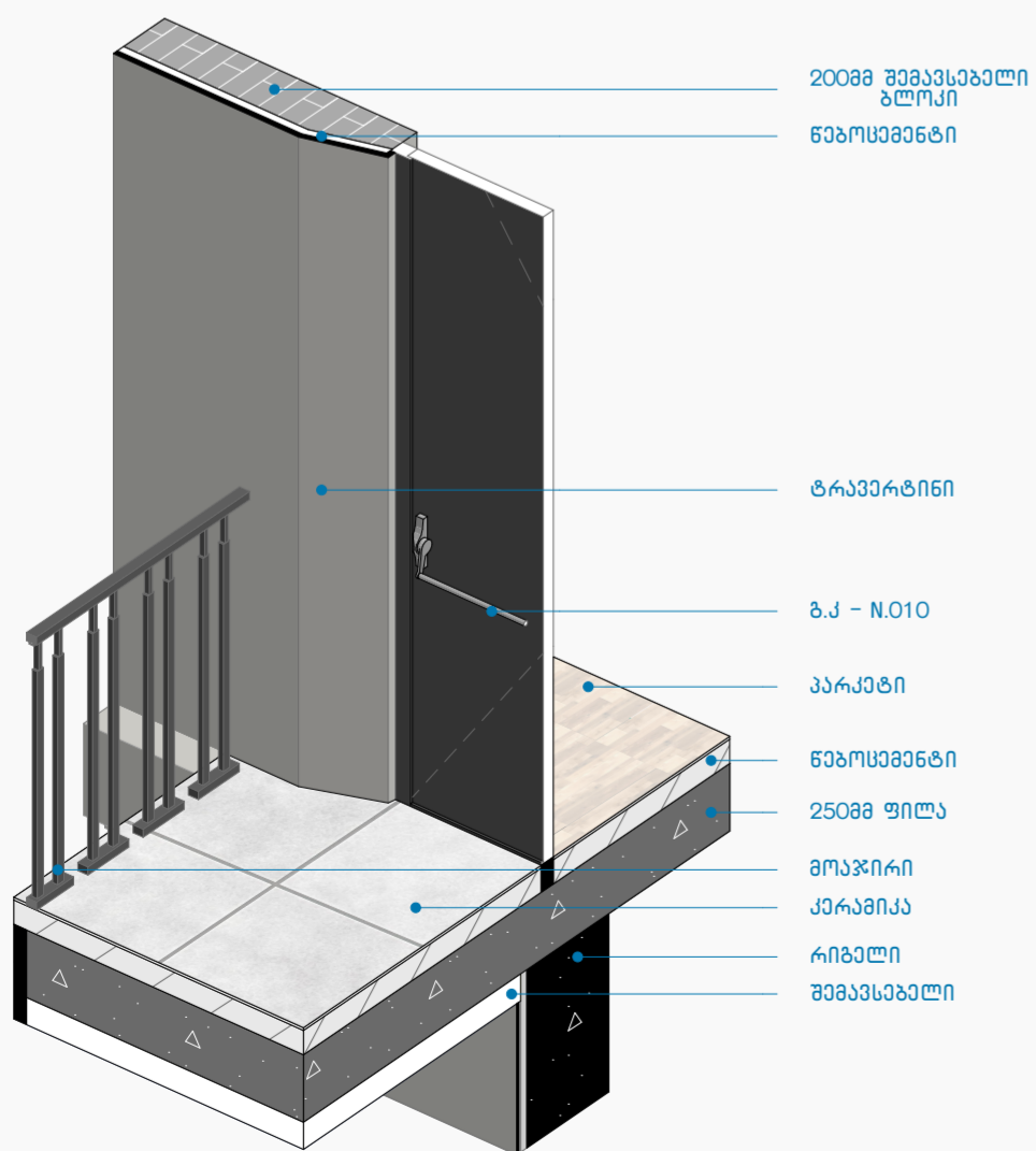
კვანძი N24 1:25
