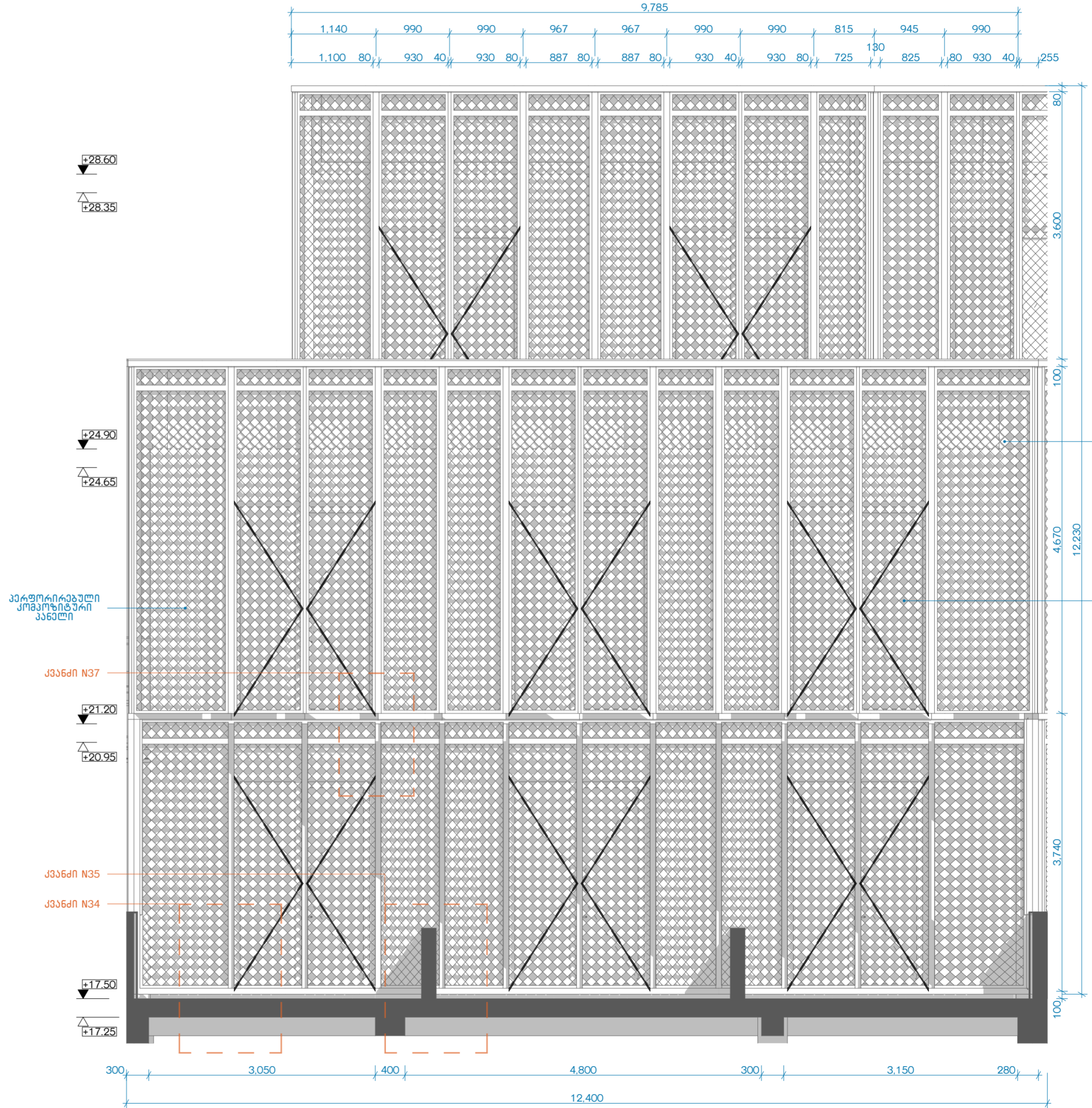
ფასადი 1-8 / ფ-21 1:50
