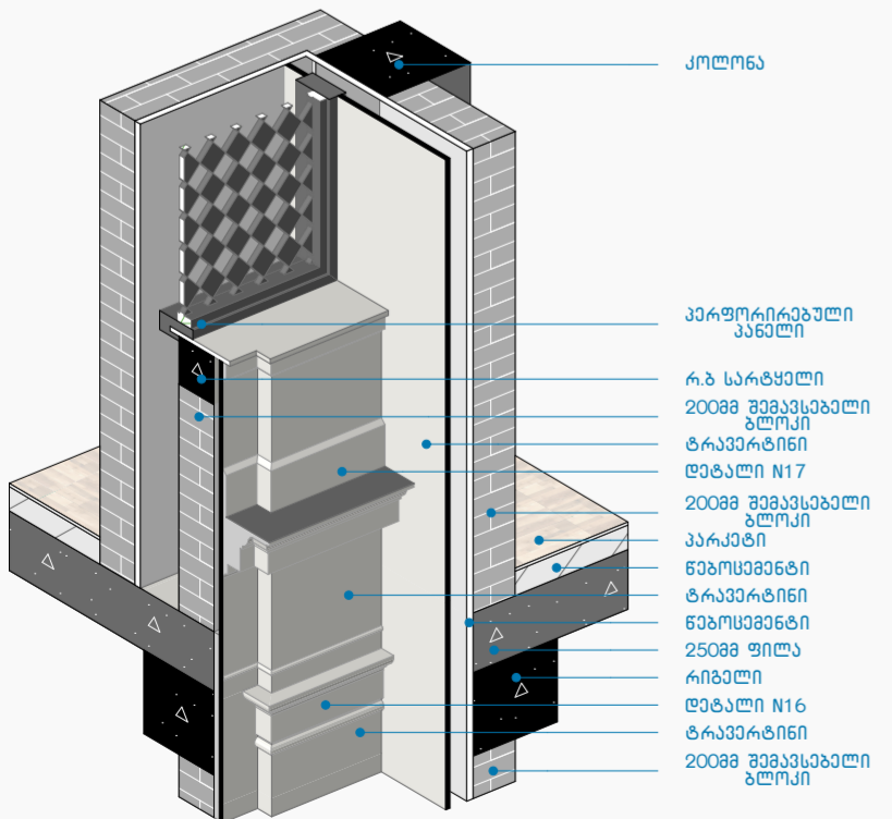
კვანძი N11 1:30
