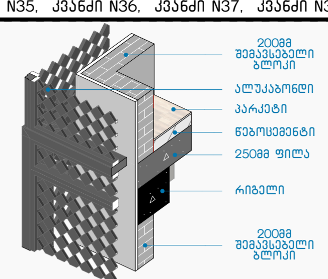
კვანძი N38 1:30
