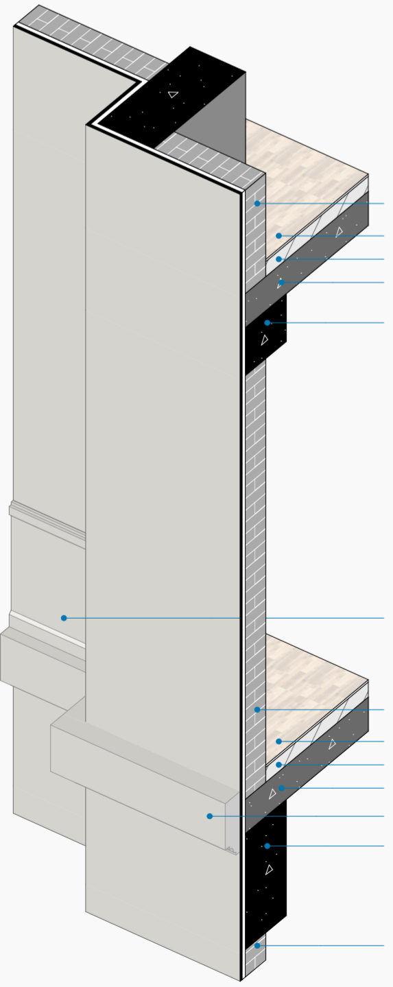
კვანძი N28 1:30
