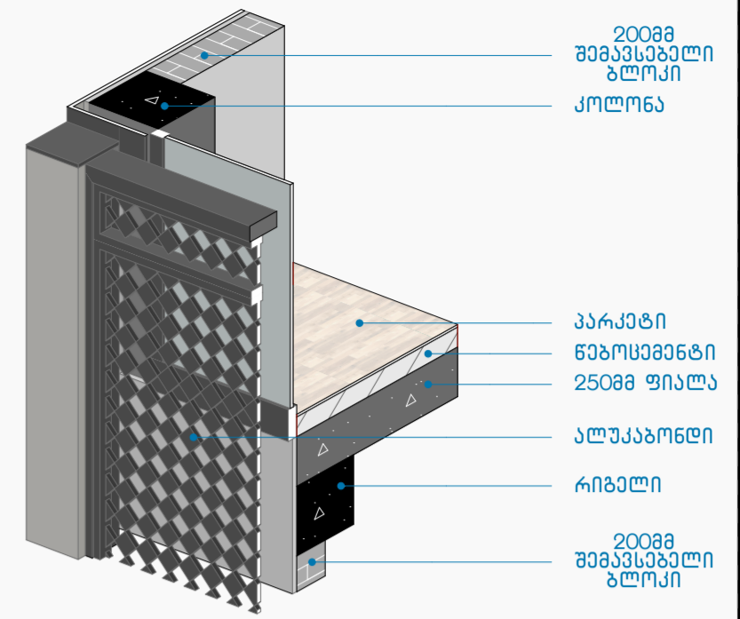
კვანძი N47 1:30
