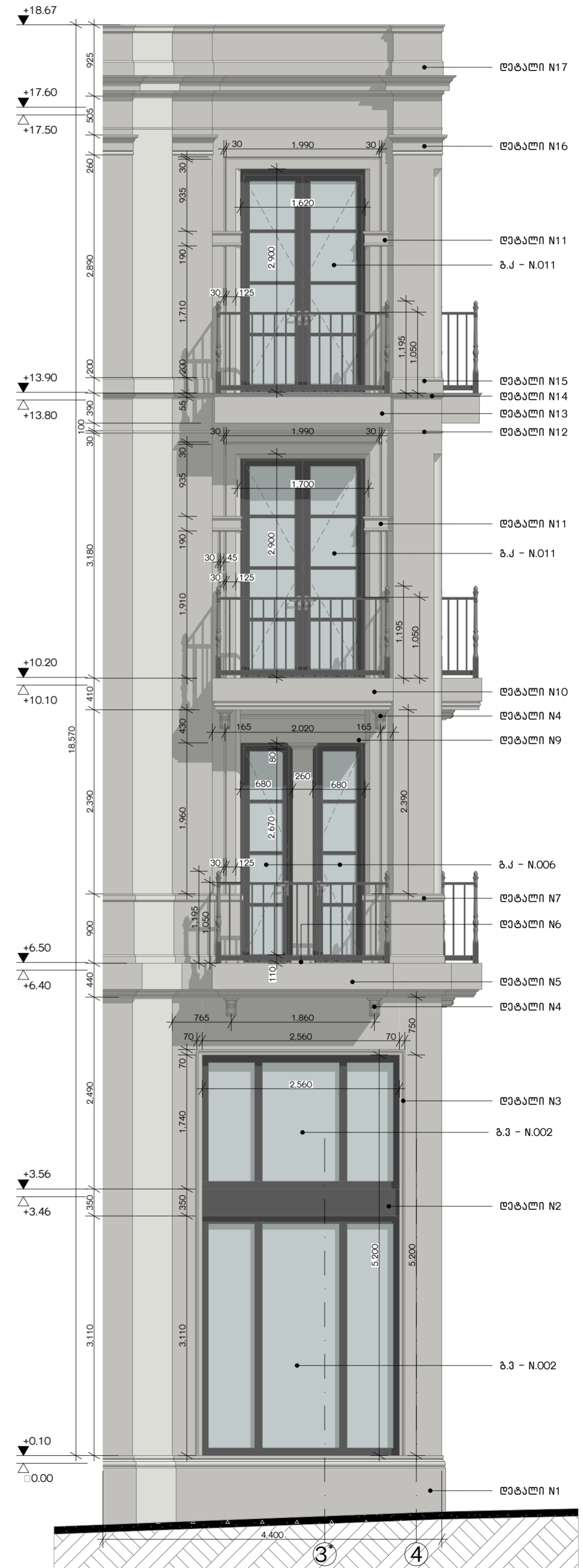
ფასადი 1-8 / ფ-7 1:50
