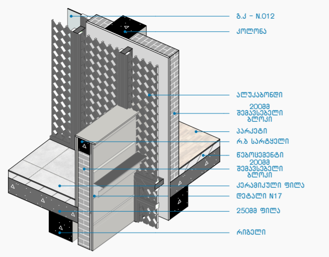
კვანძი N41 1:50
