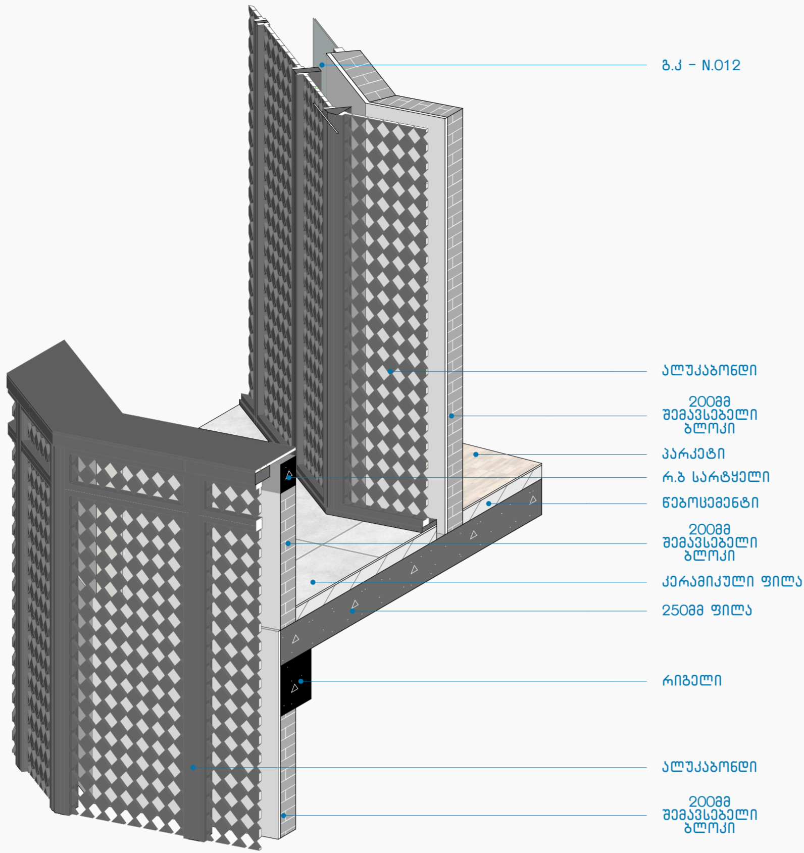
კვანძი N56
