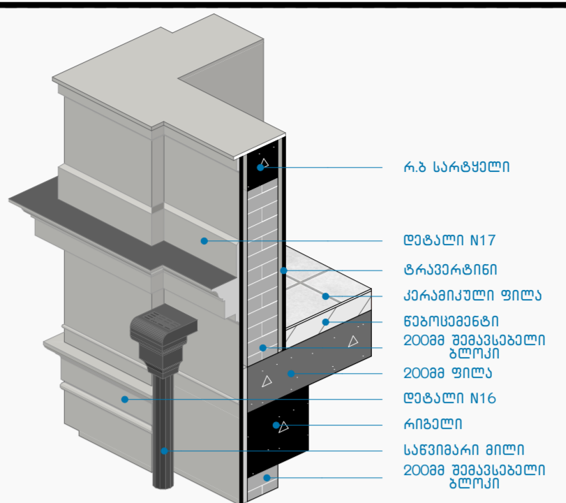
კვანძი N15 1:25
