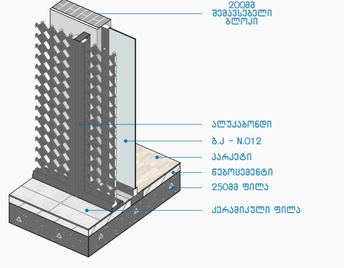
კვანძი N42 1:40
