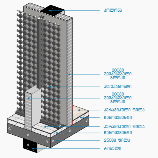
კვანძი N50 1:50
