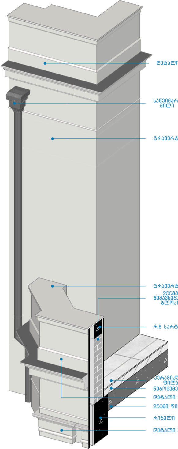
კვანძი N17 1:30
