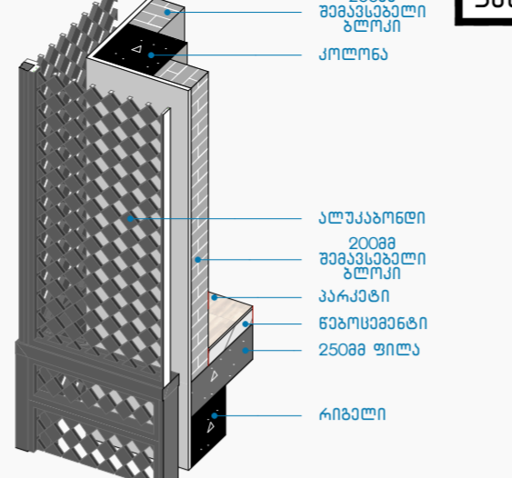
კვანძი N43 1:40
