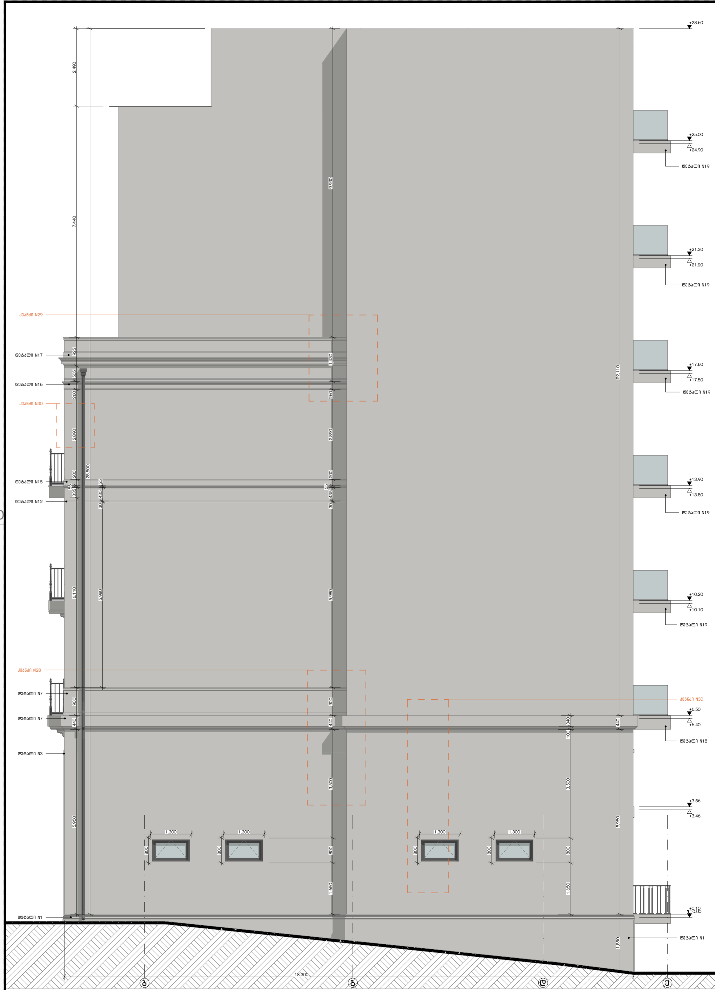
ფასადი ა-თ / ფ-18 1:75
