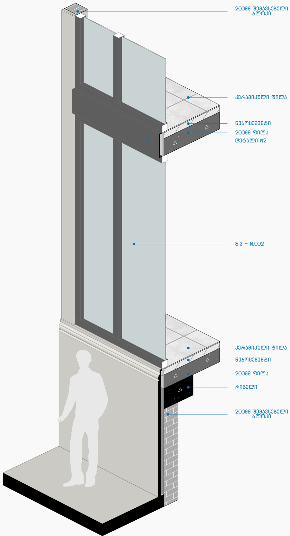
კვანძი N25 1:25
