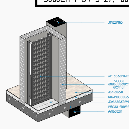
კვანძი N52 1:50
