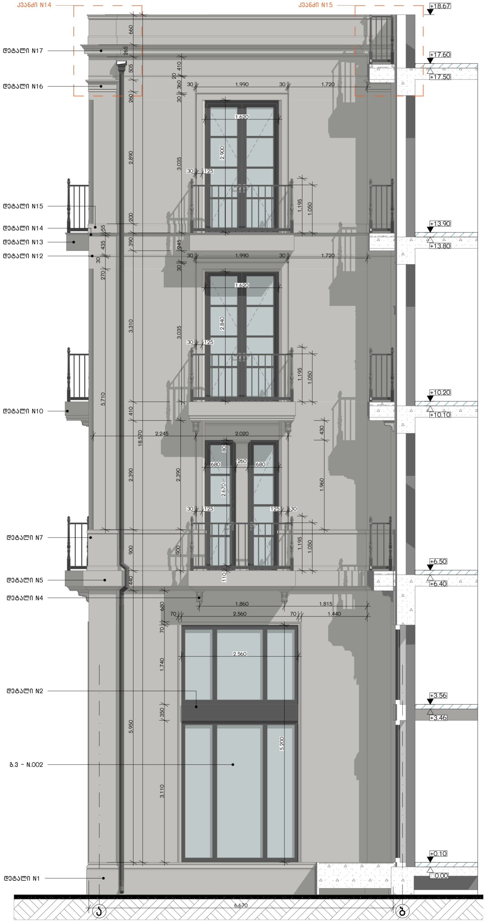
ფასადები 1-8 ღებობი / ფ-6 1:50
