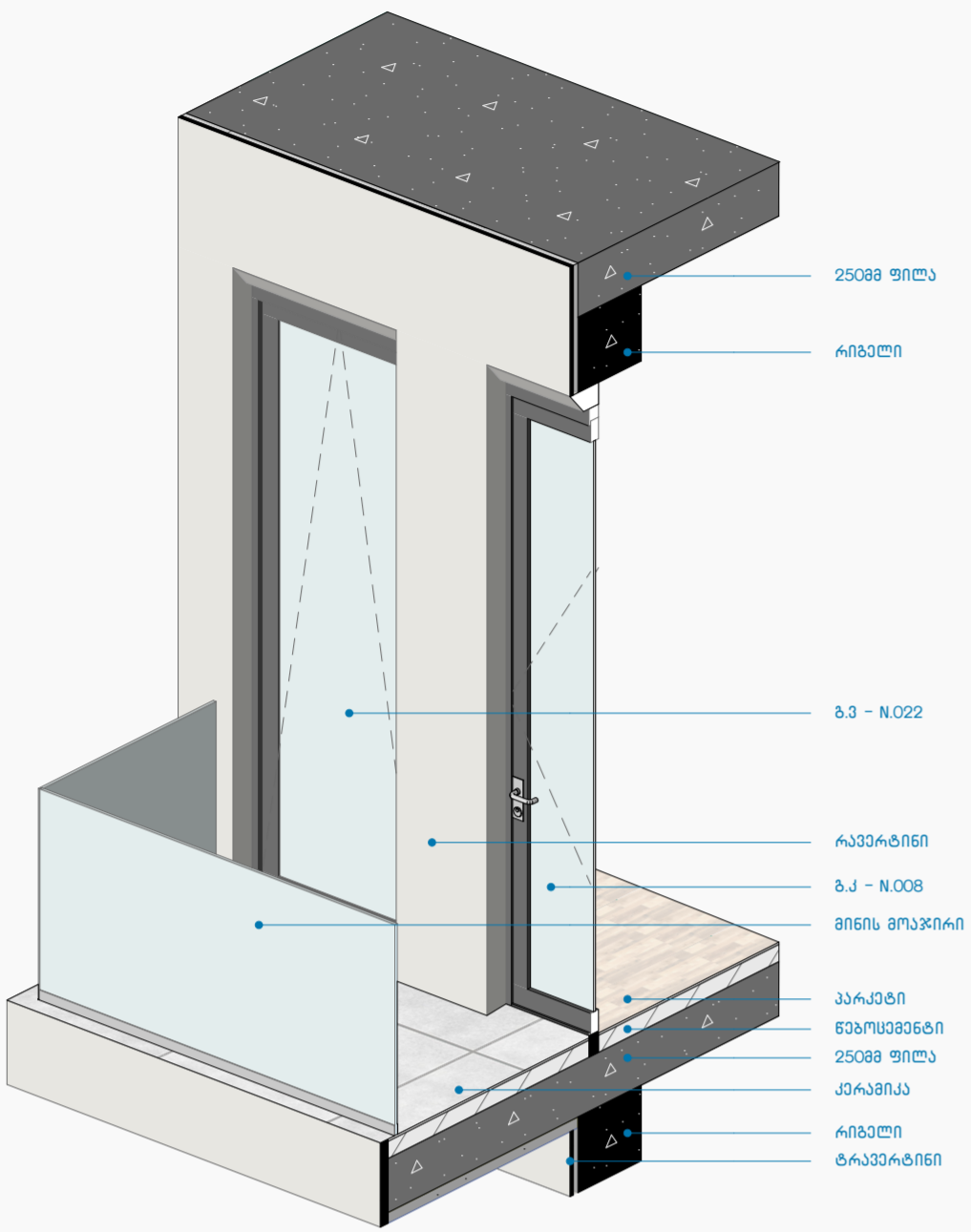
კვანძი N23
