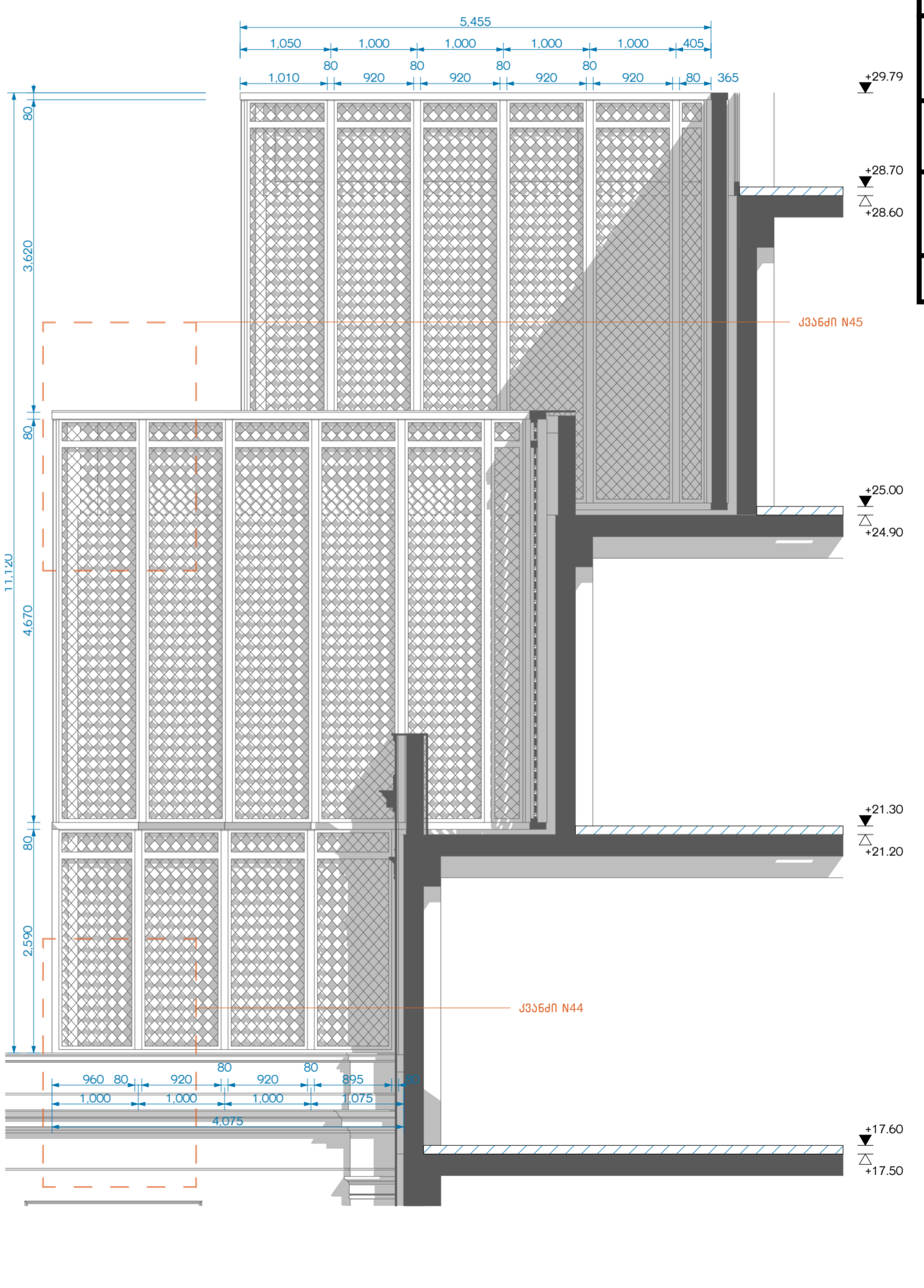
ფასადი 1-8 / ფ-24 1:50
