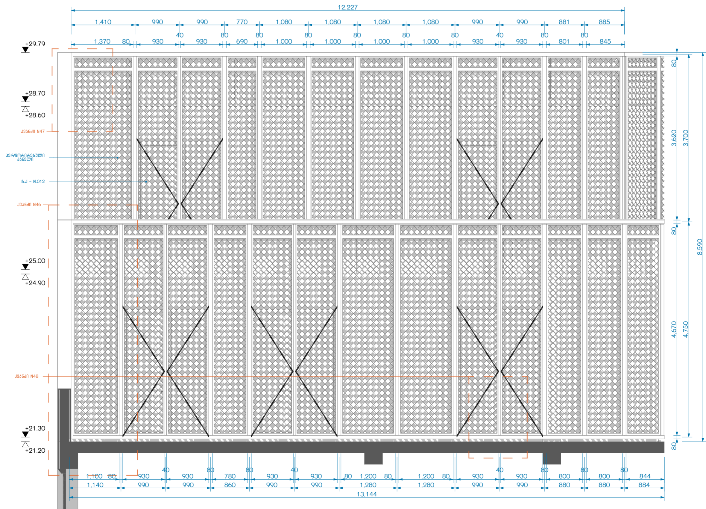
ფასალი 1-8 / ფ-29 1:50
