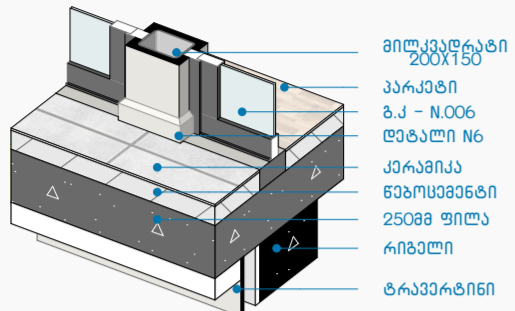
კვანძი N3 1:30
