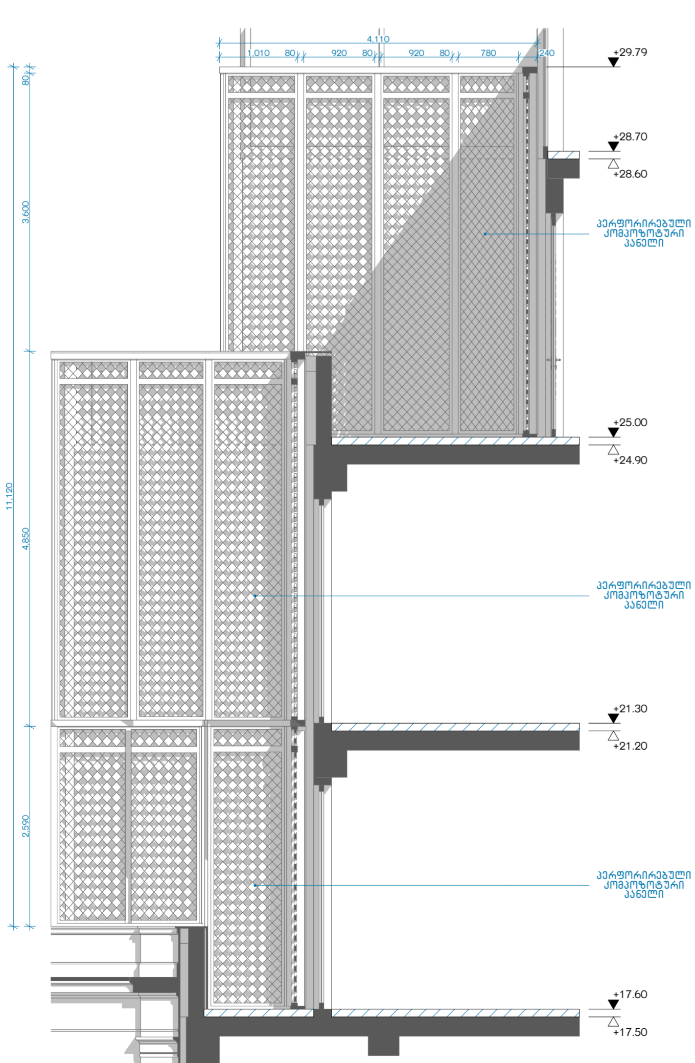
ფასადი 1-8 / ფ-20
