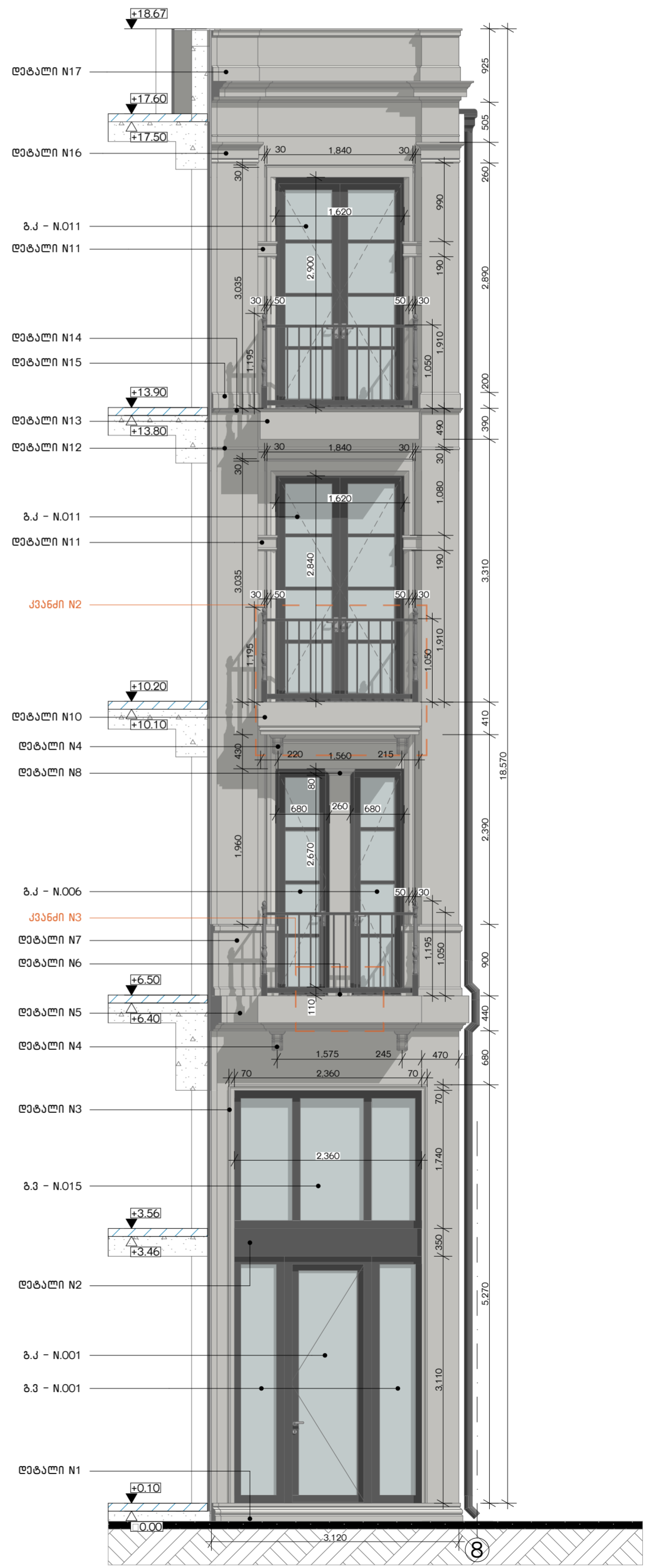
ფასადი 1-8 ლიქებში / ფ-1 1:50
