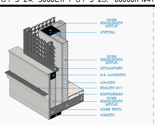
კვანძი N44 1:50
