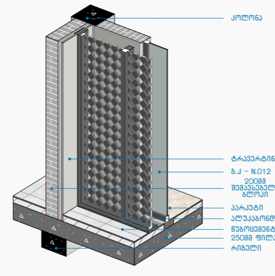
კვანძი N51 1:50
