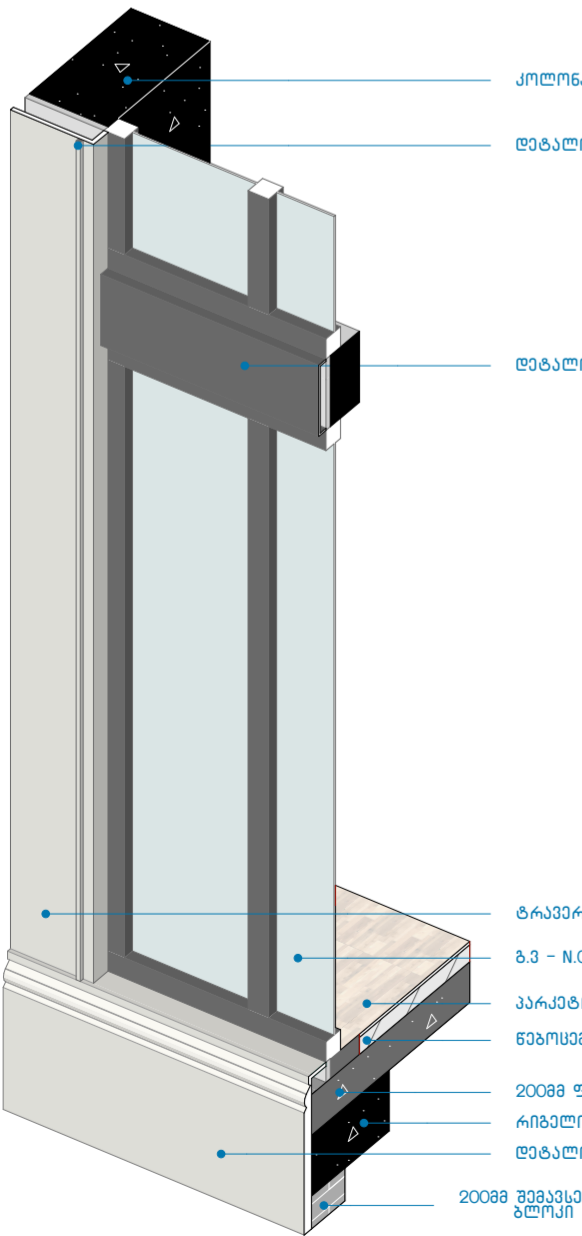
კვანძი N16 1:30
