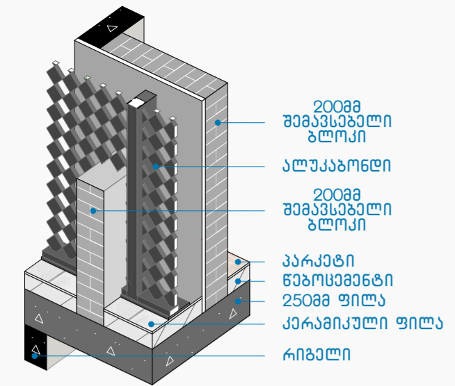
კვანძი N34 1:30
