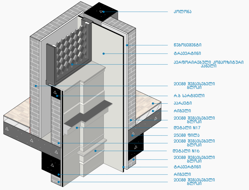
კვანძი N14 1:30
