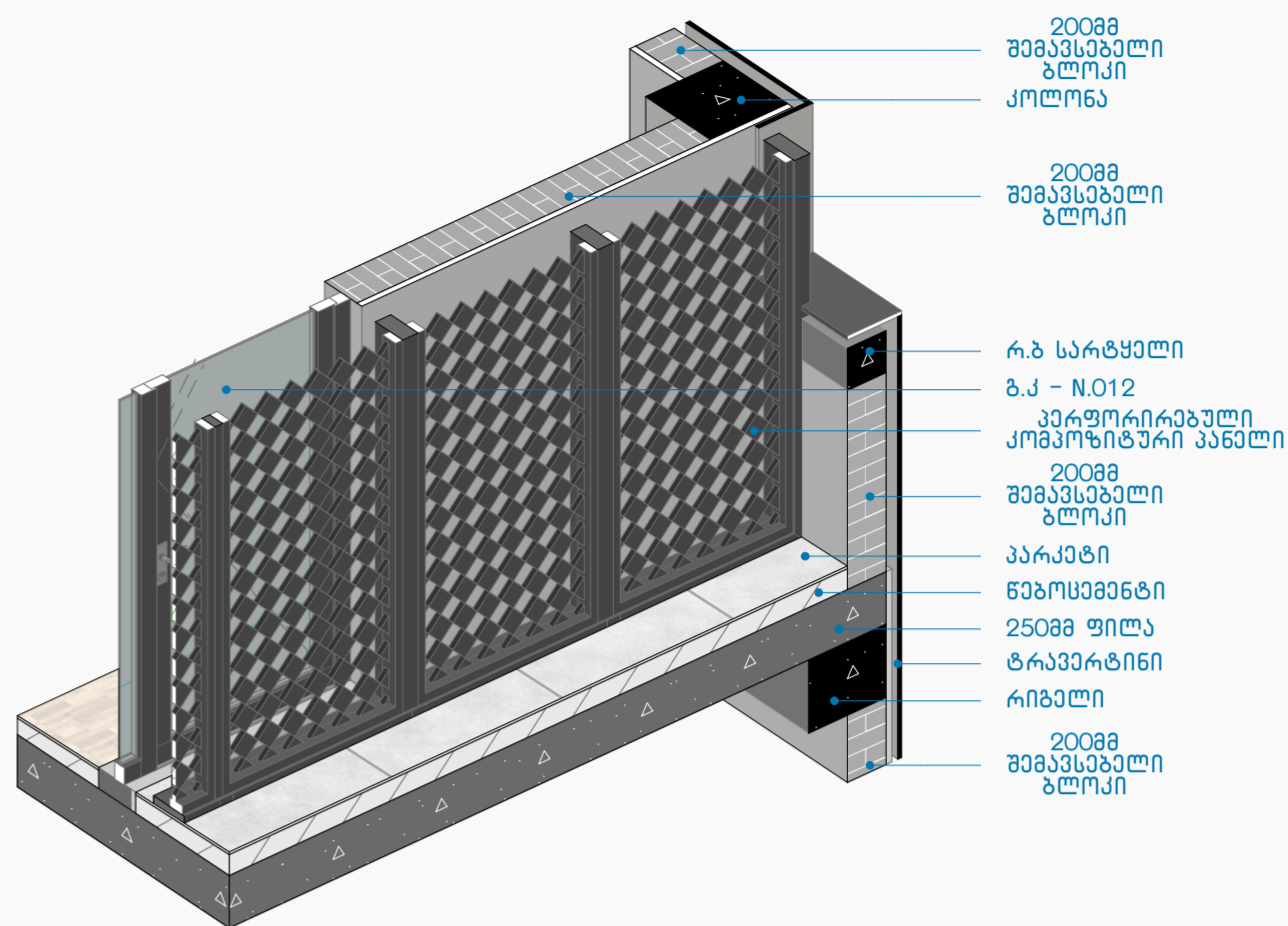
კვანძი N33
