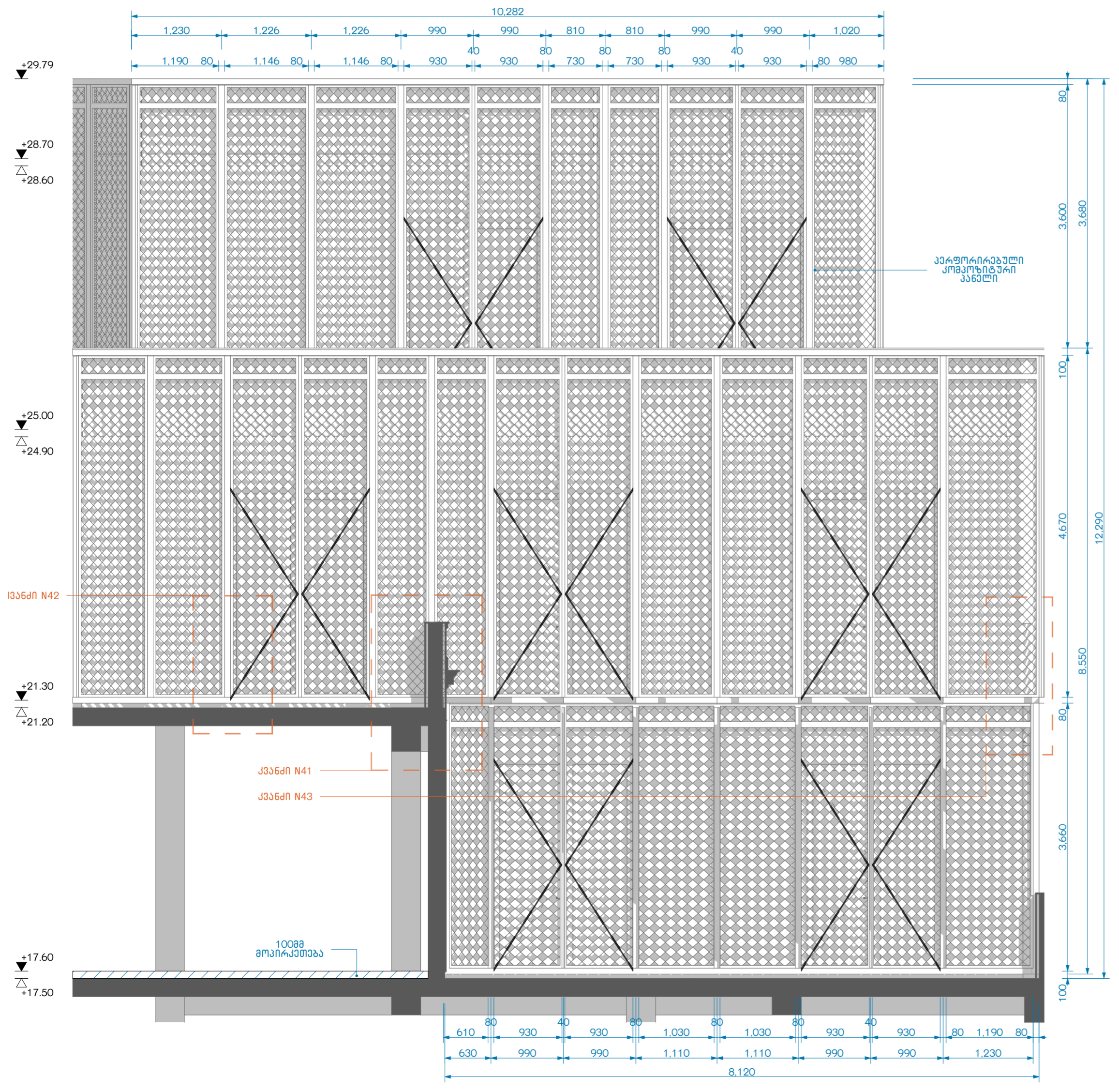
ფასადი 1-8 / ფ-25 1:50
