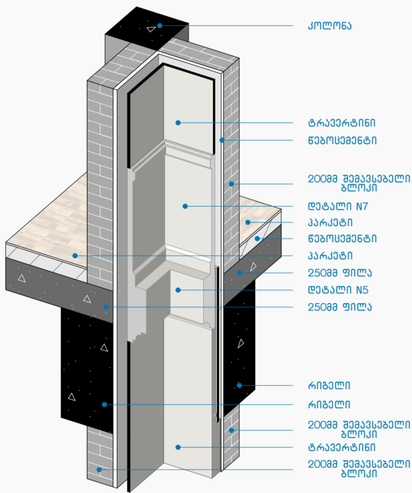
კვანძი N12 1:25
