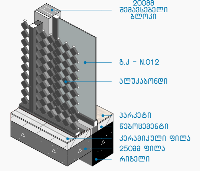
კვანძი N35 1:30
