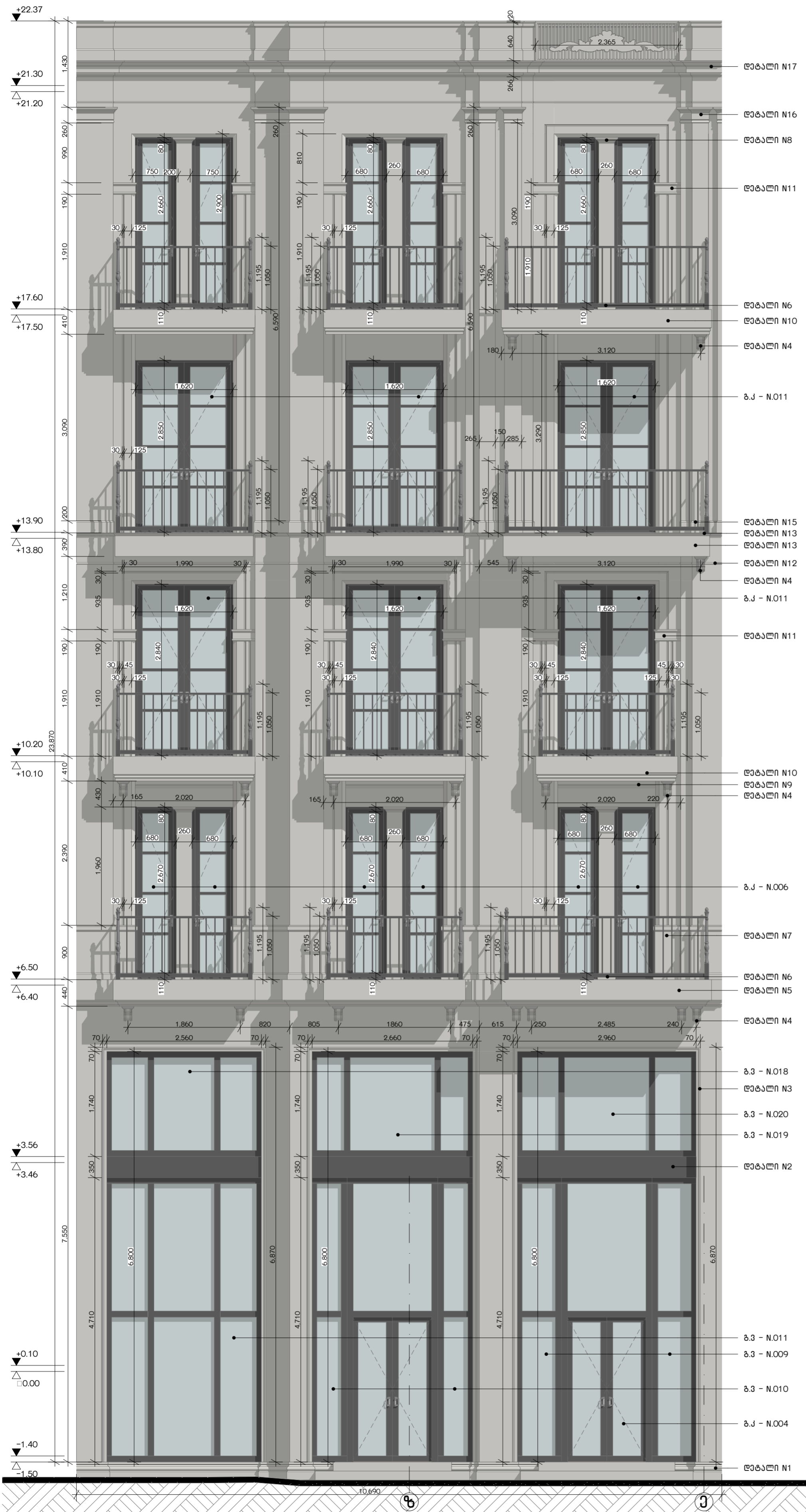
ფასალი თ-ა ლერძები / ფ-12
