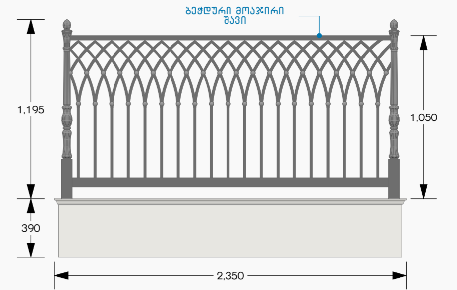
კვანძი N10 1:25
