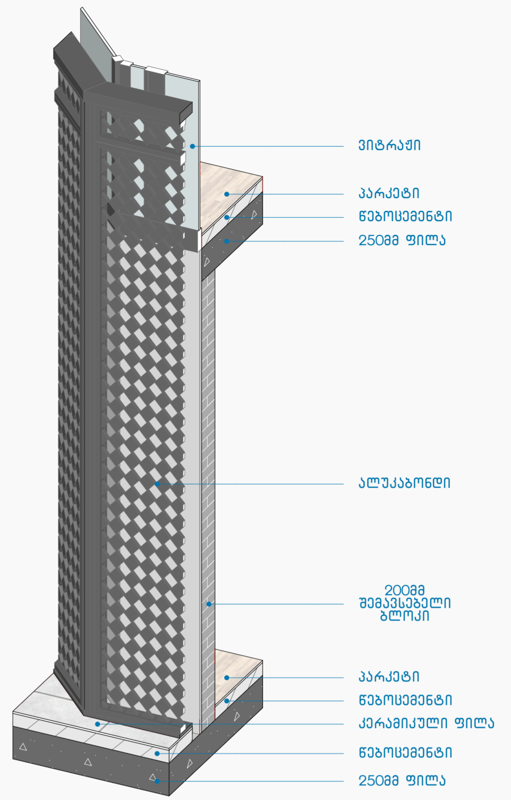
კვანძი N55
