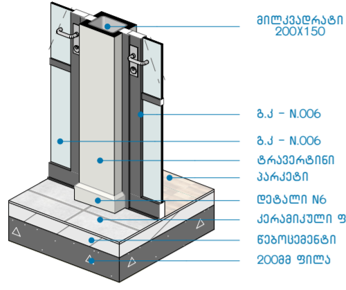
კვანძი N18 1:30
