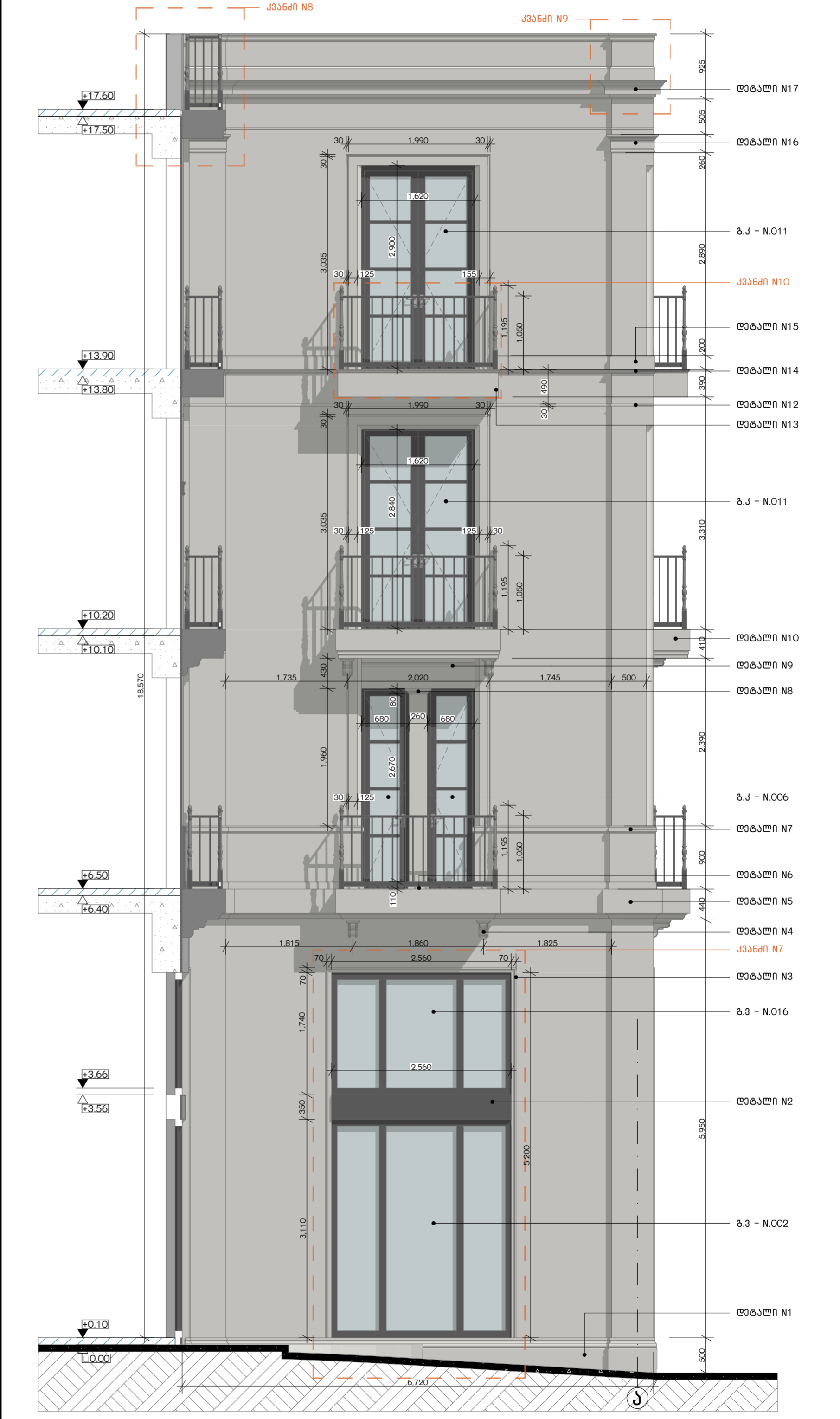
ფასადი 1-8 ლერძებში / ფ-4 1:50
