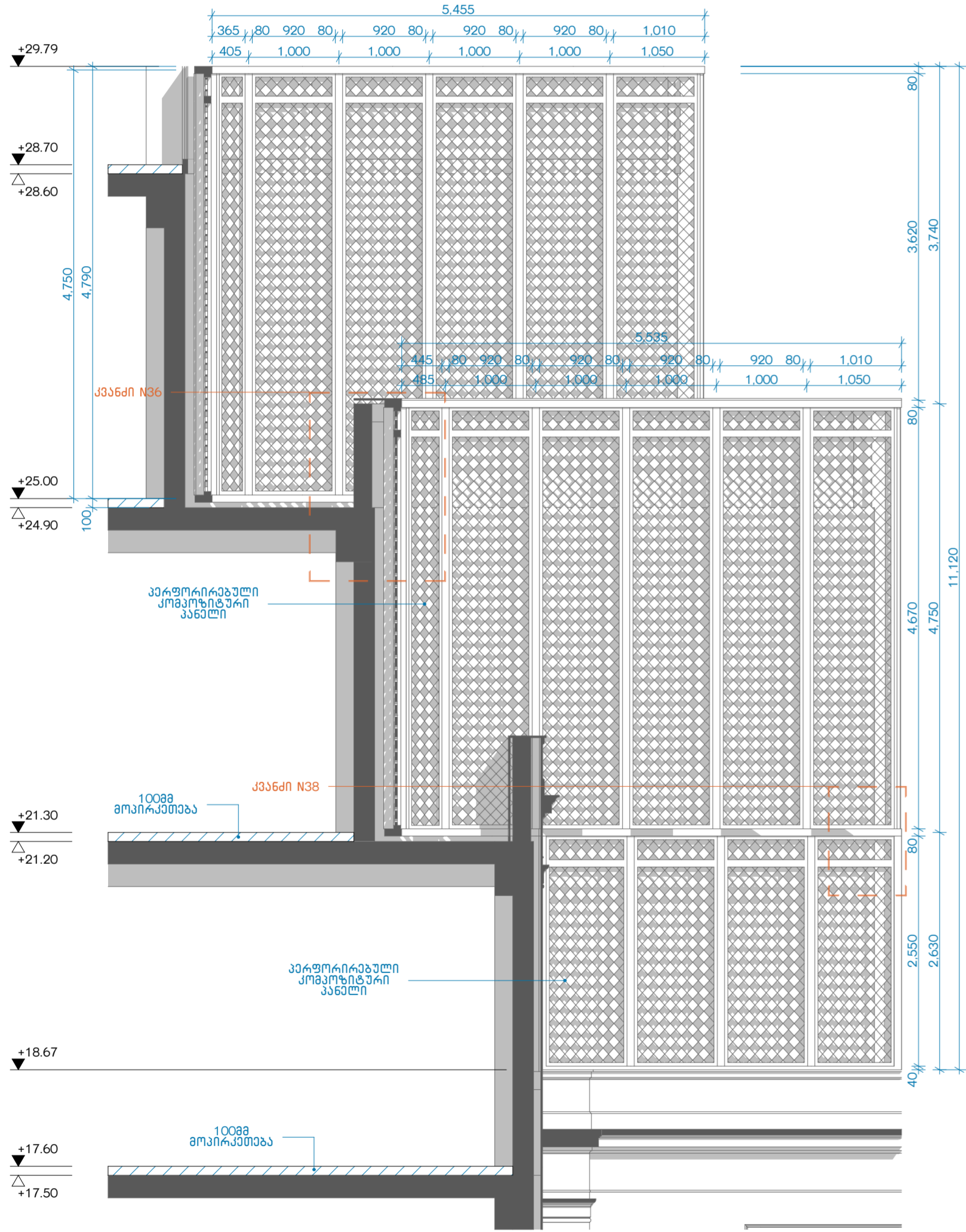
კვანძი N34 1:30
