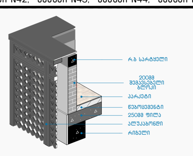
კვანძი N45 1:40
