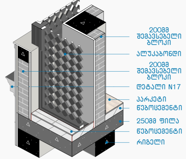
კვანძი N36 1:30
