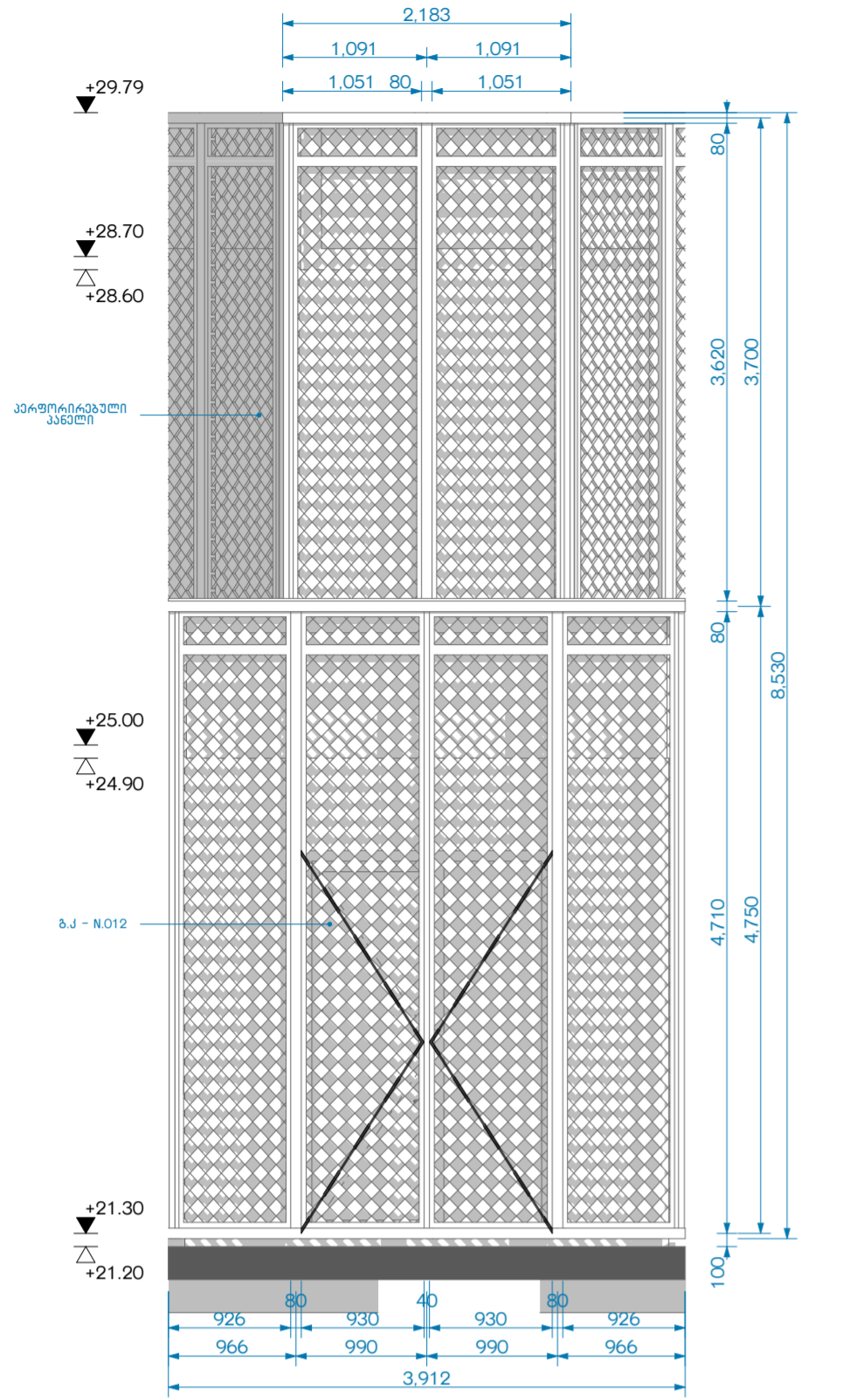
ფასალი 1-8 / ფ-28 1:50
