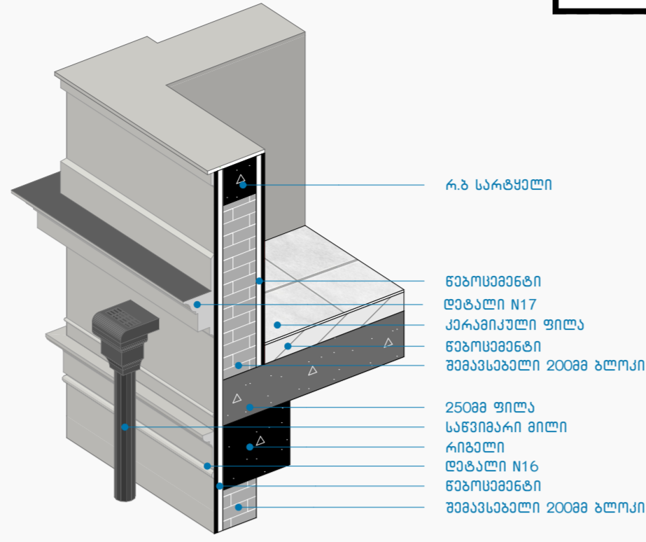
კვანძი N1 1:25
