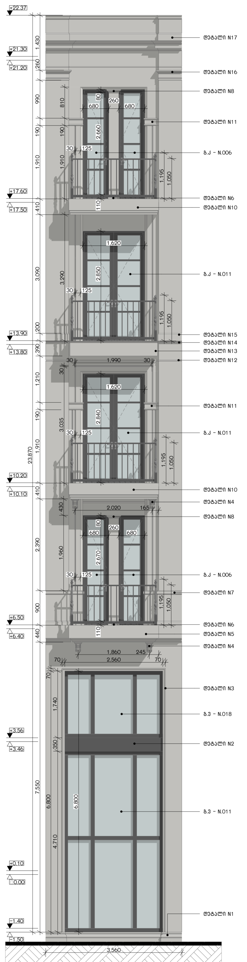
ფასალი თ-ა ლერძები / ფ-13
