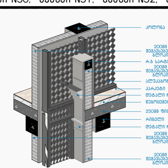
კვანძი N53 1:50
