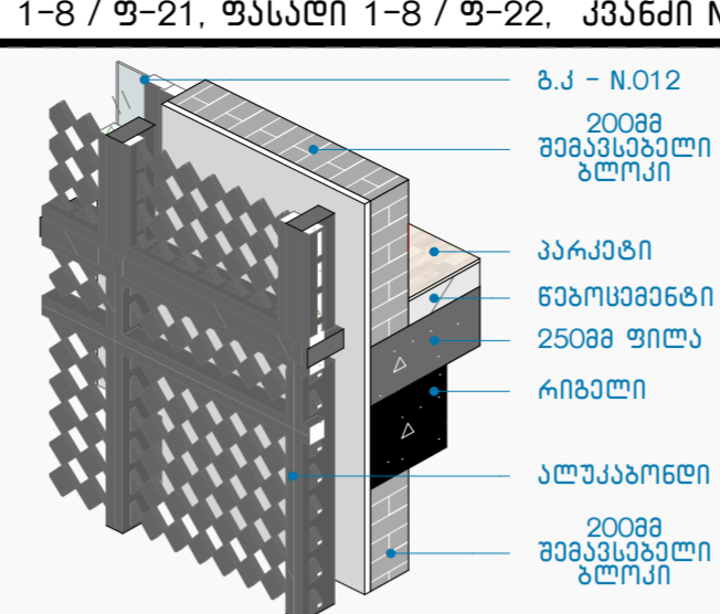
კვანძი N37 1:30
