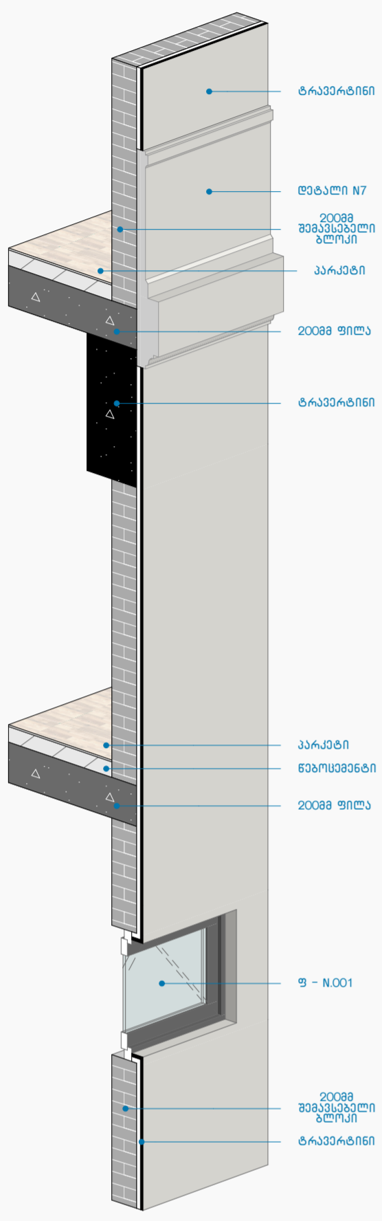
კვანძი N30 1:30
