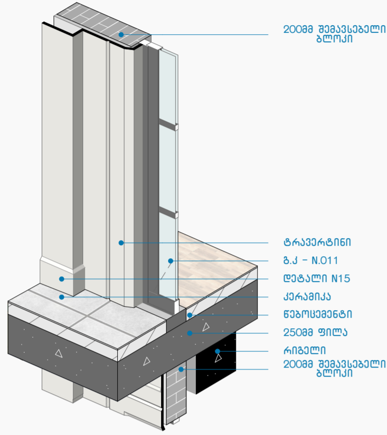
კვანძი N13 1:25
