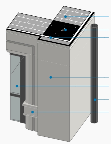
კვანძი N31 1:30
